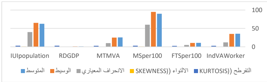
شكل رقم (١) الإحصائيات الوصفية للبيانات
