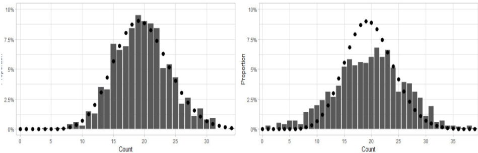
شكل رقم (٦) اختبار التكامل المشترك
